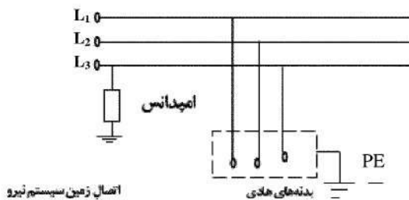
شکل ۵ پ سیستم TT
