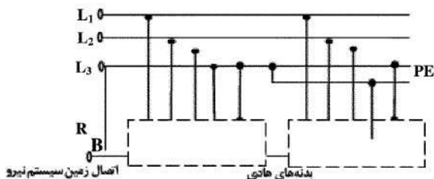
شکل ۲ پ سیستم TN-C-S با هادی مشترک حفاظتی-خنثی در بخشی از سیستم.
