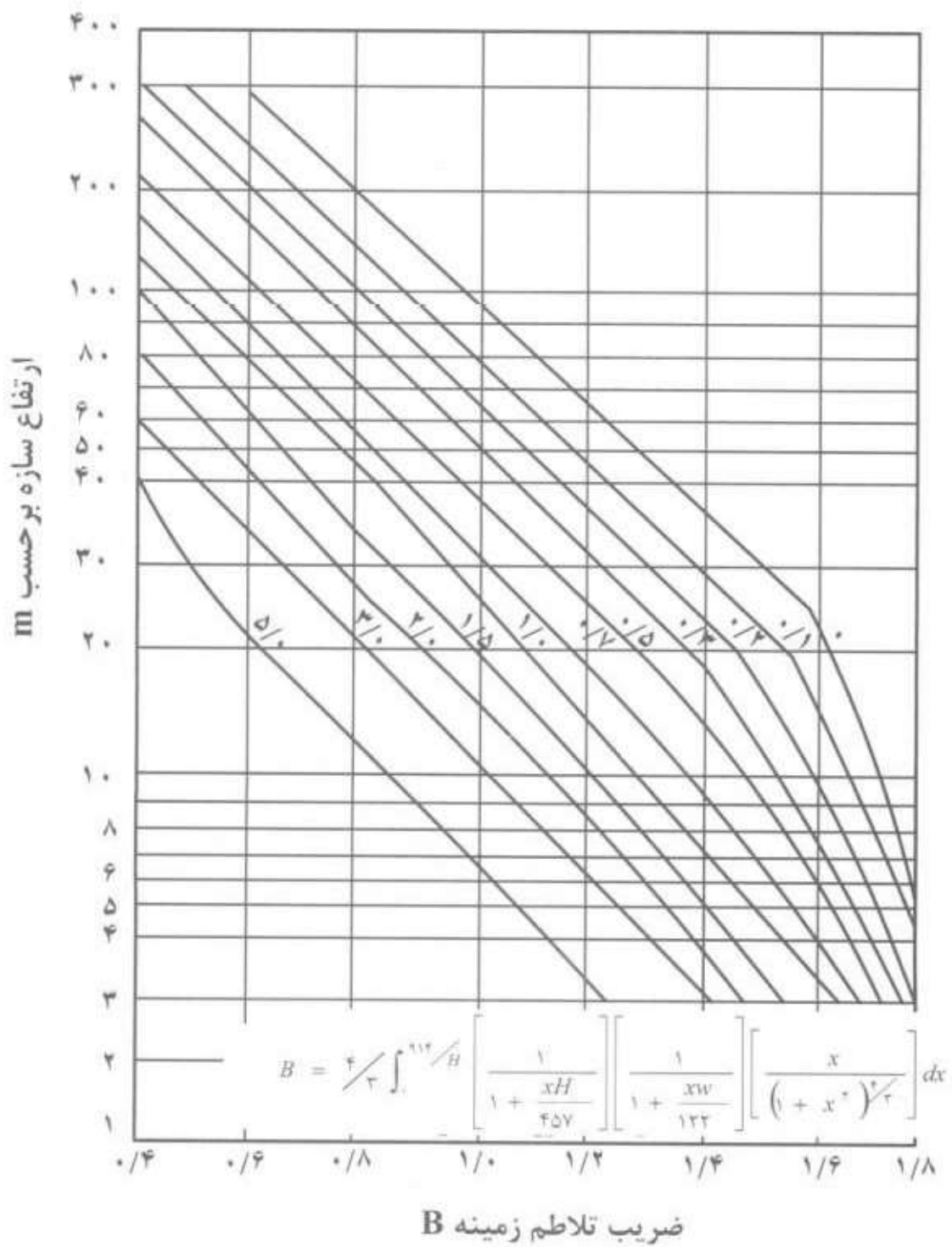
شکل پ-۶-۲-۲ ضریب تلاطم زمينه بعنوان تابعی از عرض و ارتفاع سازه
