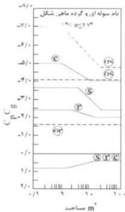
شکل ۱۰-۶-۵ ضرایب ترکیبی بیشینه فشار - جهش باد خارجی، C_p C_q ، روی بام‌های شیروانی تک دهانه و چند شیبه با شیب 7^\circ یا بیشتر برای طراحی اجزای و پوسته خارجی
