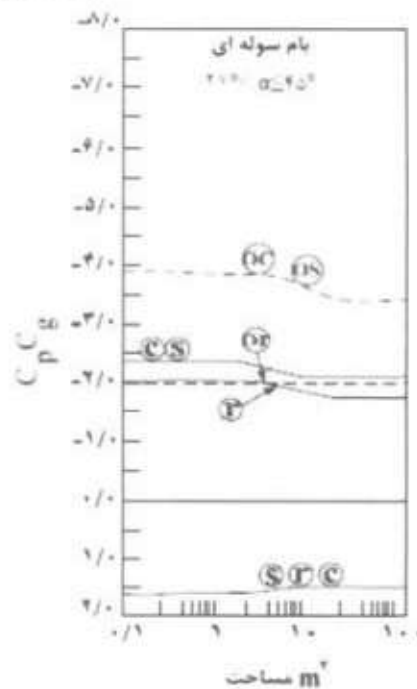
شکل ۱۰-۶-۵ ضرایب ترکیبی بیشینه فشار - جهش باد خارجی، C_p C_q ، روی بام‌های شیروانی تک دهانه و چند شیبه با شیب 7^\circ یا بیشتر برای طراحی اجزای و پوسته خارجی
