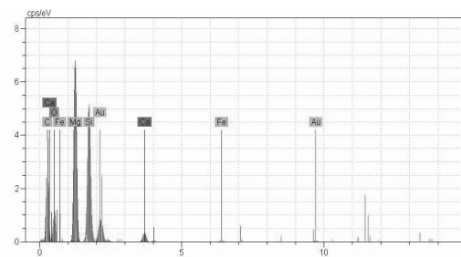
شکل ۲: طیف EDXA الیاف کریزوتایل در نمونه هوا به روش میکروسکوپ الکترونی روبشی.
