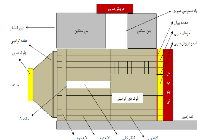
شکل (۱): ساختار ستون حرارتی راکتور تهران
