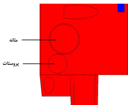
شکل (۱): نمای جانبی لگن در یک برش از فانتوم در نقطه x=0.5 و موقعیت پروستات و مئانه در آن
