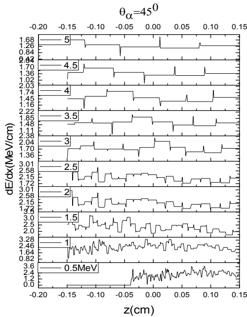
شکل (۶): پاسخ آشکارساز به ذرات آلفا با زاویه 45^\circ .
