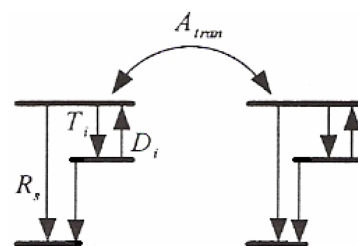
شکل (۲): مسیرهای مجاز الکترون برای بازترکیب شدن مستقیم و غیر
