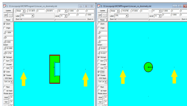
شکل (۶): محل قرارگیری کره‌های کوچک برای اندازه‌گیری پرتوگیری حول سیستم.
