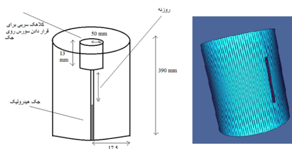
شکل (۳): ساختار و ابعاد محفظه‌ی سربی برای محدود کردن
