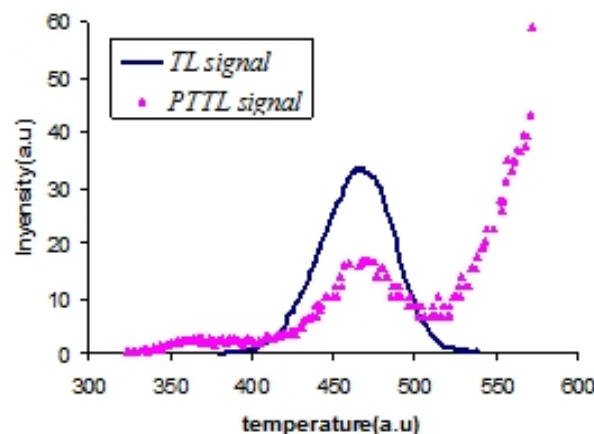
شکل ۲: منحنی شدت TL و PTTL بر حسب دما به‌ازای دز گامای ۰/۱ mGy
