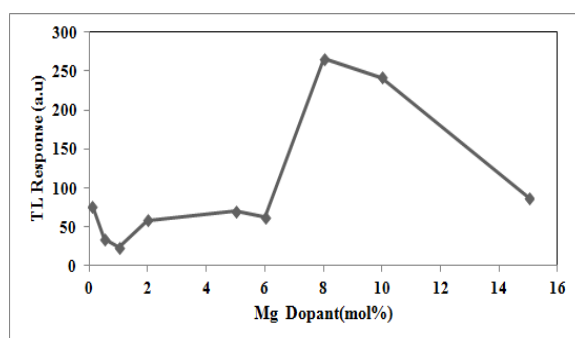
شکل ۴: نمودار تأثیر میزان ناخالصی منیزیم در حساسیت نانوذرات لیتیوم تترا بورات آلائیده با منیزیم
