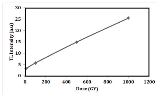
شکل ۵: نمودار پاسخ ترمولومینسانس نانوذرات لیتیوم تترابورات آلاینده با منیزیم نسبت به پرتو گاما
