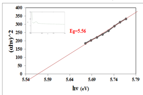
شکل ۷: نمودار جذب نانوذرات لیتیوم تترابورات آلاینده با منیزیم و محاسبه گاف انرژی از روی نمودار
