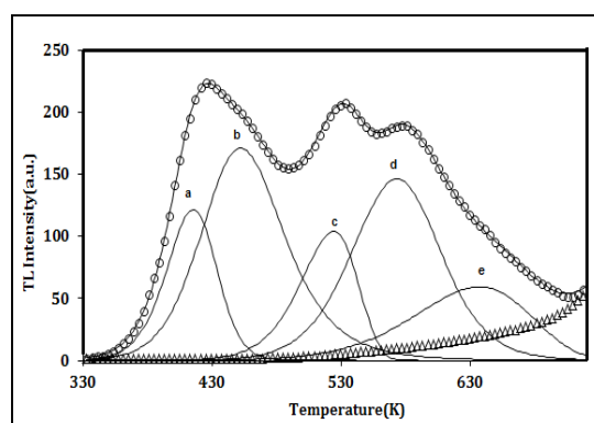
شکل ۳: منحنی تابش ترمولومینسانس برازش شده نانوذرات لیتیوم تترا بورات آلائیده با منیزیم
