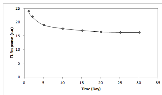
شکل ۶: نمودار محوشدگی نانوذرات لیتیوم تترابورات آلاینده با منیزیم
