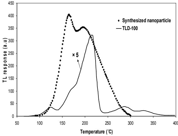
شکل (۸): نمودار مقایسه حساسیت ترمولومینسانس نانو ذرات \text{CaF}_2:\text{Ti} با \text{TLD-100} (\text{LiF}:\text{Mg,Cu,P})
