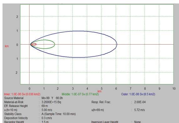
شکل (۶): میزان انتشار دز در اطراف راکتور برای کلاس A با سرعت باد ۵ m/s
