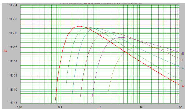
شکل (۳): TEDE محاسبه شده در فواصل مختلف (Sv) برای تمامی کلاس‌های جوی با سرعت باد ۲ m/s
