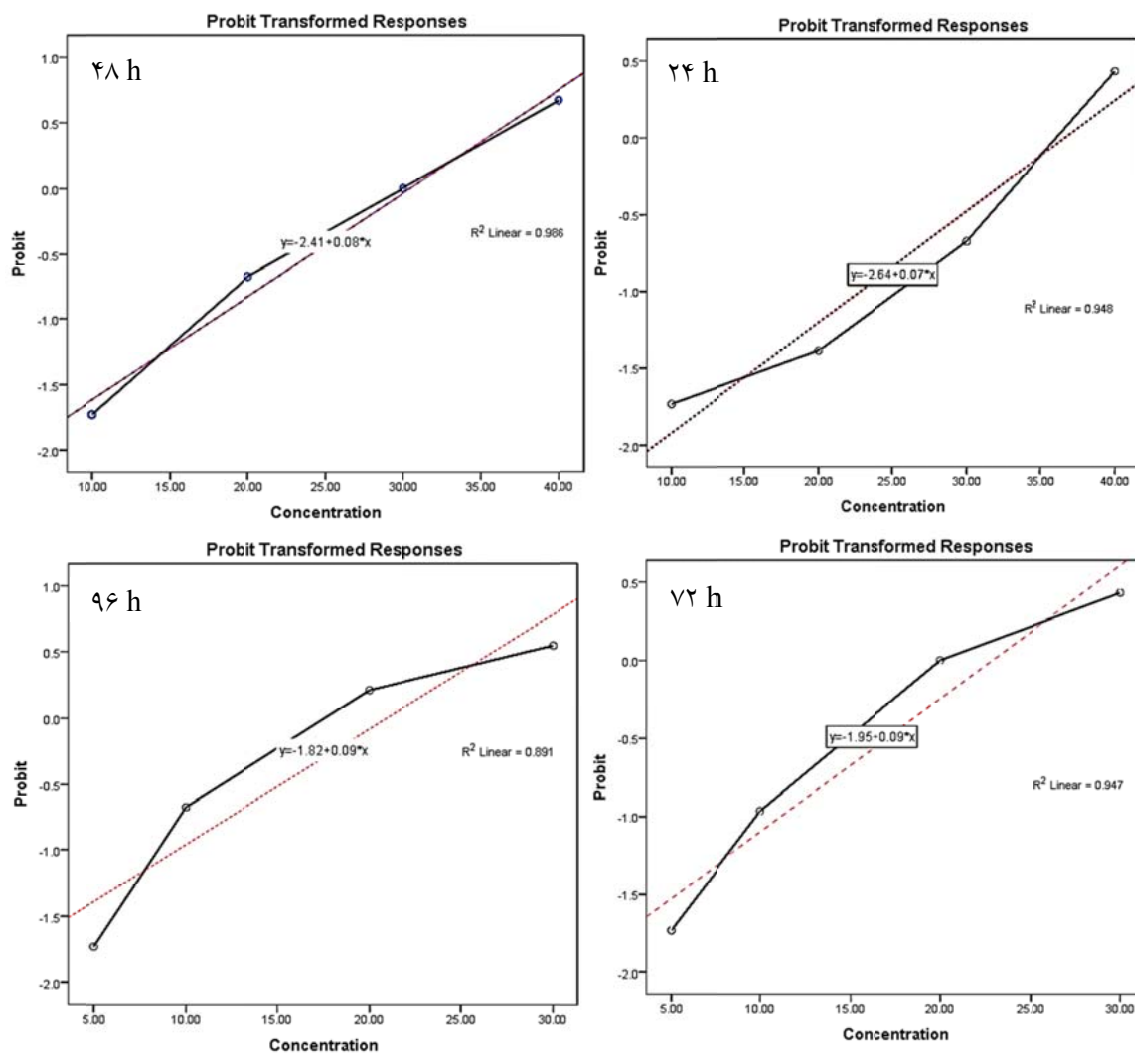
نمودار ۲- آنالیز Probit و رگرسیون خطی بین غلظت سم گلایفوزیت و روند مرگ و میر ماهی کپور معمولی در بازه‌های زمانی ۲۴ تا ۹۶ h
