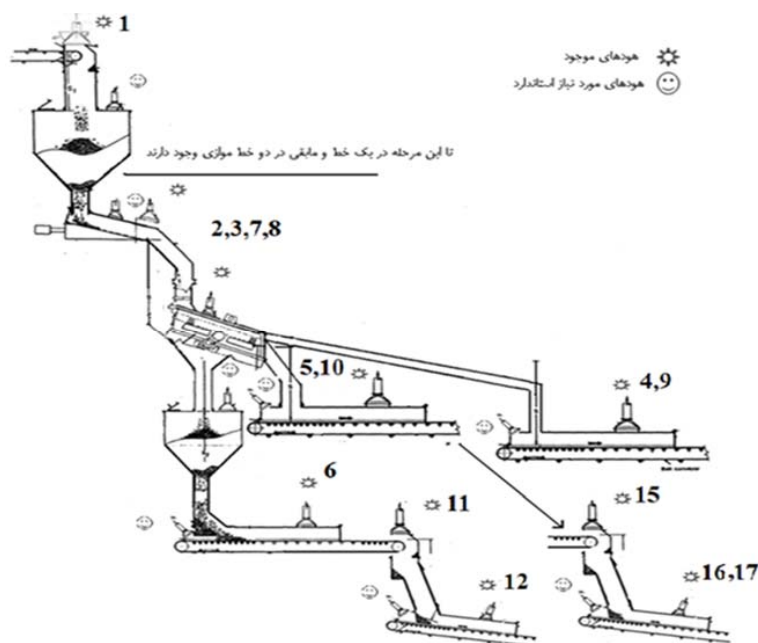
شکل ۲. فرایند غربال و انتقال مواد در واحد، منابع اصلی آلودگی، هودهای موجود و هودهای مورد نیاز (۴)
