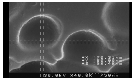
شکل ۳. نمونه‌ای از اندازه نانوذرات اکسید نیکل در بستر رزین
