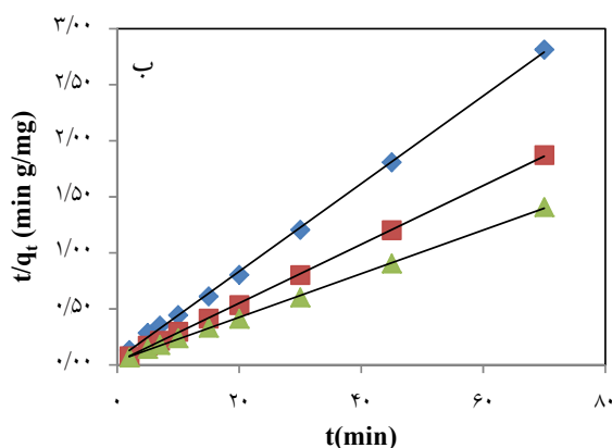
نمودار ۵- جذب سطحی رنگ متیل اورانژ توسط نانوذرات مغناطیسی نیکل بر اساس مدل سینتیکی (الف) شبه درجه اول و (ب) شبه درجه دوم
