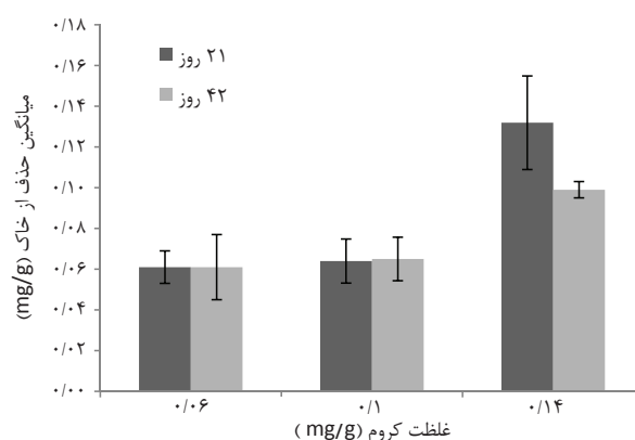
شکل ۱- میانگین کروم موجود در خاک بر حسب غلظت‌های اولیه در زمان‌های مختلف مورد بررسی
