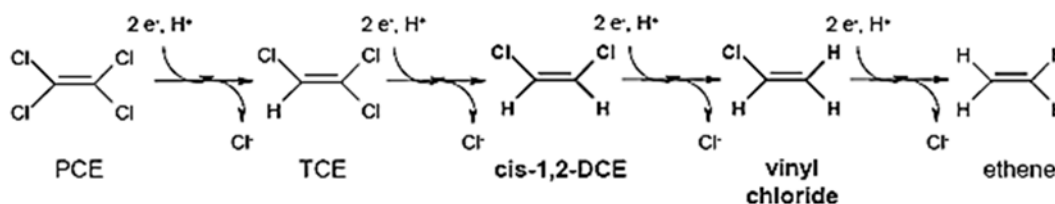
شکل ۱- توالی واکنش های کلرزدایی تتراکلرواتیلن توسط عامل احیا کننده یا دهنده الکترون [USEPA; 2004]
