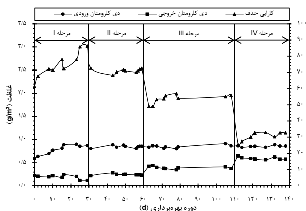
شکل ۲: عملکرد و راندمان کلی بیوراکتور HBCB در حذف دی کلوامان از فاز گازی
