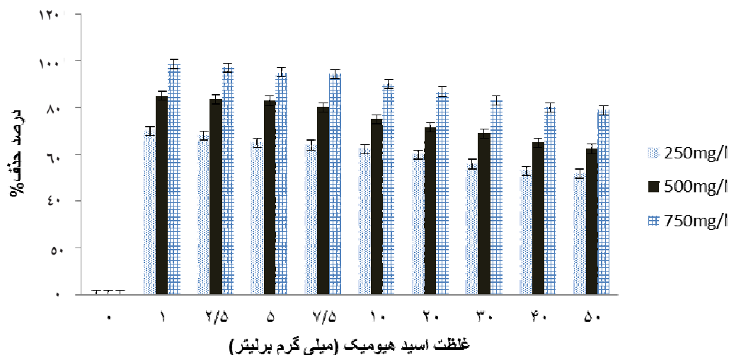
شکل ۴: تاثیر غلظت‌های مختلف نانوذرات اکسید آهن پوشش داده با سیلیس بر غلظت‌های مختلف اسید هیومیک در pH ۵/۱ و زمان ۹۰ min
