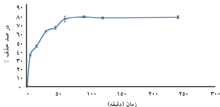
شکل ۳: بازده حذف اسید هیومیک در زمان‌های مختلف، pH ۵/۱، غلظت اولیه اسید هیومیک ۱۰ mg/L و غلظت جاذب (۵۰۰ mg/L)
