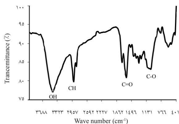
شکل ۲- الف: طول موج FTIR پوست سبز گردو از ۴۰۰ تا cm^{-1}
