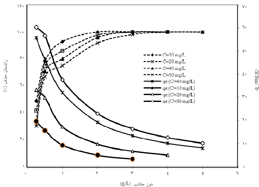
شکل ۵: تأثیر دوز جاذب (پوست سبز گردو) در راندمان و ظرفیت جذب در حذف فنل (غلظت های اولیه ۱۰-۵۰ mg/L)
