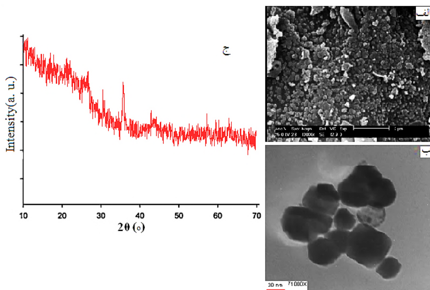
شکل ۲: تصویر SEM جاذب(الف)، تصویر TEM جاذب (ب)، الگوی پراکنش اشعه ایکس مربوط به \text{Fe}_3\text{O}_4 (ج).
