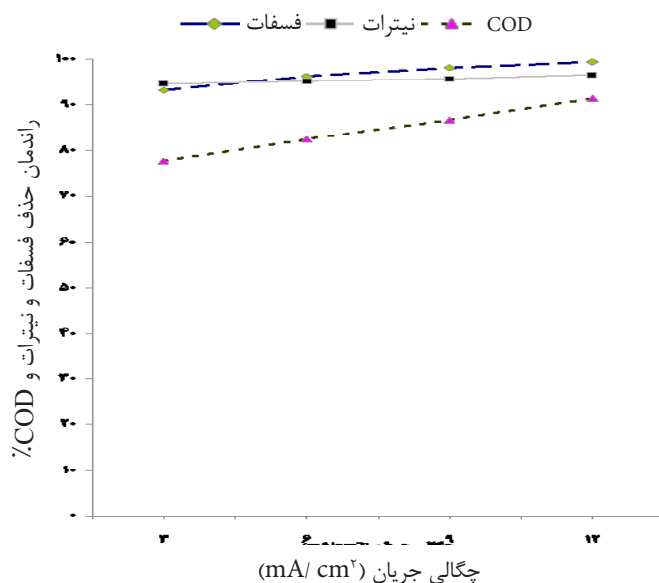
شکل ۷: مقادیر حذف فسفات، نیترات و COD با استفاده از الکترود آهنی و تغییر شدت جریان الکتریکی چگالی جریان (mA/cm 2 )
