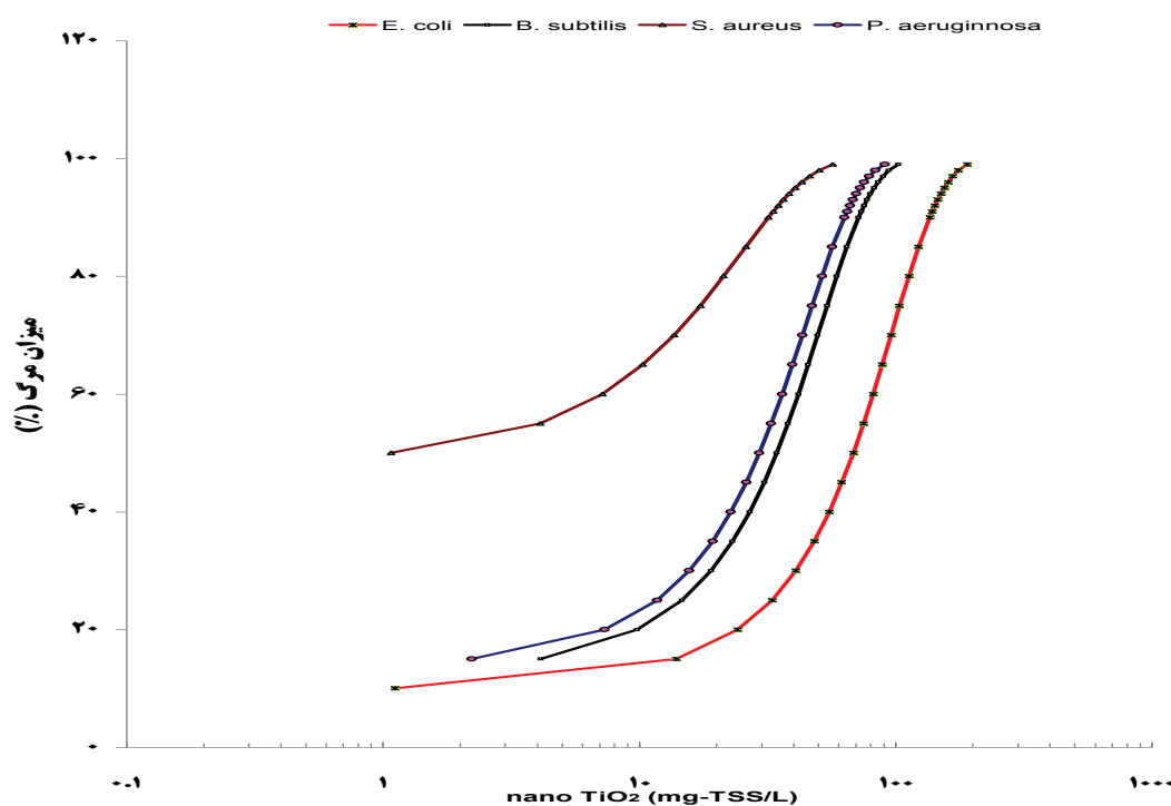
شکل ۱: دوز پاسخ باکتری‌های مختلف در اثر مواجهه با نانوذرات TiO_2
