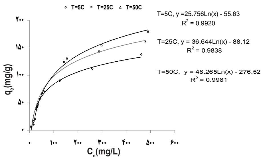
شکل ۴: ایزوترم‌های جذب
