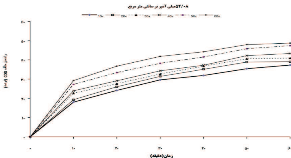
شکل ۲: راندمان تغییرات COD از شیرابه در زمان مختلف pH=7.52 و هدایت الکتریکی 52/0.8 (ms/cm)
