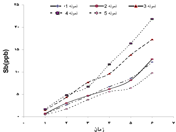
شکل ۶: تغییرات غلظت آنتیموان در زمان‌های مختلف در شرایط نگهداری در دمای 80^{\circ}\text{C}
