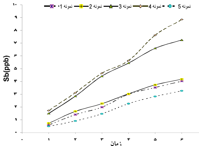
شکل ۵: تغییرات غلظت آنتیموان در زمان‌های مختلف در شرایط نگهداری در دمای 65^{\circ}\text{C}
