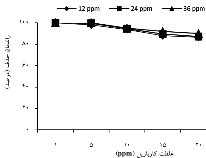
شکل ۴: منحنی درصد کارایی حذف سم کارباریل بر حسب غلظت ورودی آن به سیستم و تغییرات غلظت PAC در پایلوت PAC
