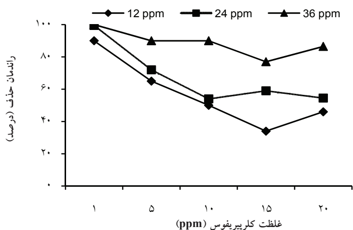
شکل ۳: منحنی درصد کارایی حذف سم کلرپیرفوس بر حسب غلظت ورودی آن به سیستم و تغییرات غلظت PAC در پایلوت PAC
