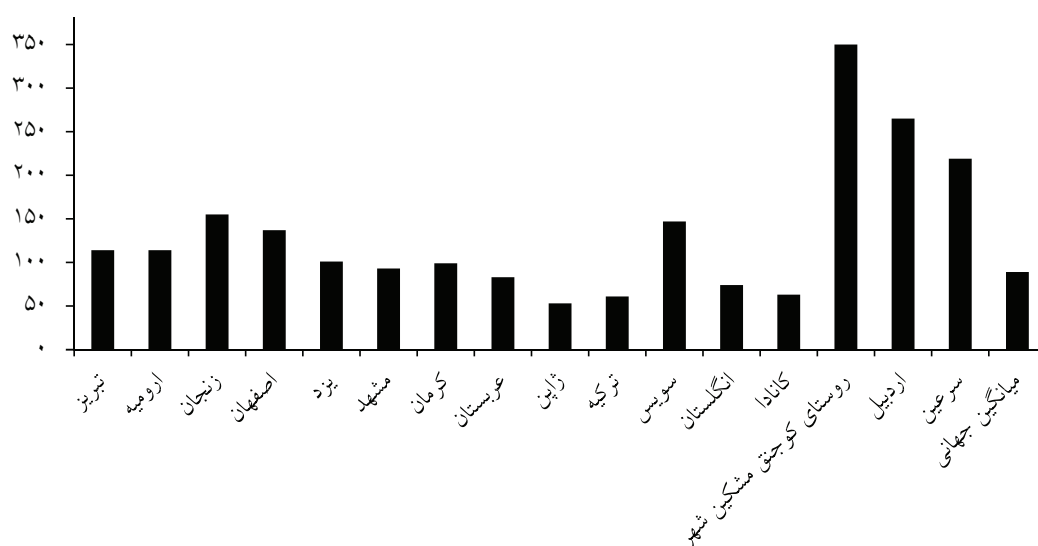
شکل ۳: نمودار مقایسه ای آهنگ دوز (نانو سیورته در ساعت) گزارش شده از ایران و جهان (۳، ۸، ۹، ۱۳، ۱۷، ۱۸، ۲۰، ۲۴، ۲۷-۲۹)
