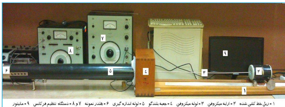
شکل ۱. لوله امپدانس مدل ۴۰۰۲ و اجزای تشکیل دهنده آن جهت تعیین ضریب جذب صوتی.
