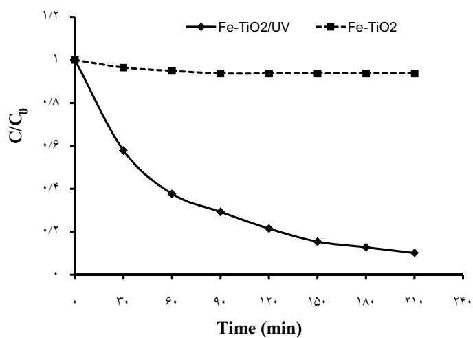
شکل ۸: تأثیر جذب سطحی \text{Fe}^{3+} -TiO 2 بر روی فنل: \text{Fe}^{3+} -TiO 2 = ۰/۵ g/L، pH = ۳، C_0 = ۱۰ mg/L
