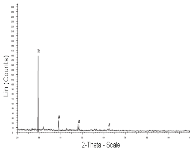
شکل ۳: الگوی پراش پرتو X: \text{Fe}^{3+}/\text{TiO}_2 = 0.34 (at %)
