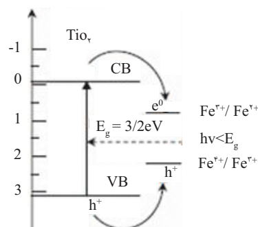
شکل ۱: تصویر شماتیکی انتقال بار الکتریکی از \text{TiO}_2 برانگیخته
