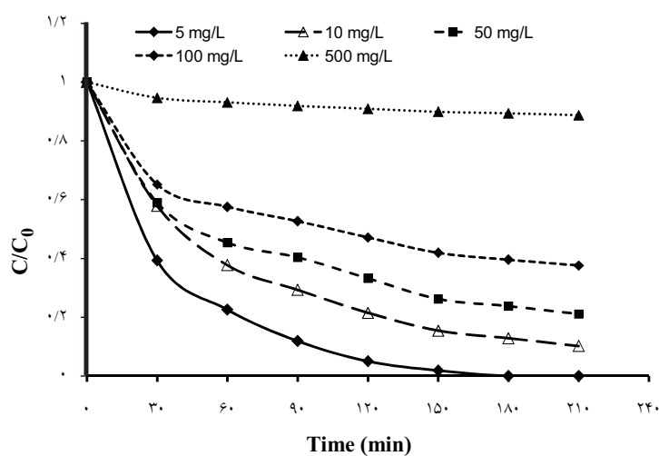
شکل ۷: تأثیر غلظت اولیه فنل در تجزیه فتوکاتالیستی: \text{Fe}^{3+} -TiO 2 = ۰/۵ g/L، pH = ۳
