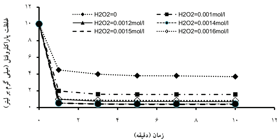
شکل ۲: تاثیر H_2O_2 بر کارایی حذف پاراکلروفنل توسط فرایند شبه فتوتون ( Fe^0=0/0.002mol/L , pH=4 , Time=5 min )
