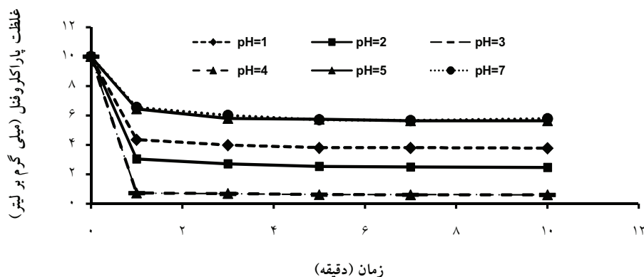
شکل ۱: تاثیر pH بر کارایی حذف پاراکلروفنل توسط فرایند شبه فتوتون ( H_2O_2=0/0.002mol/L , Fe^0=0/0.002mol/L , Time=5 min )
