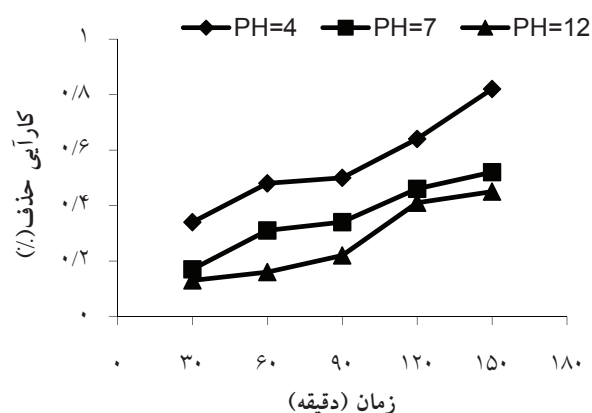
شکل ۷: رابطه pH با میزان حذف فسفر به وسیله نانو زئولیت Y
