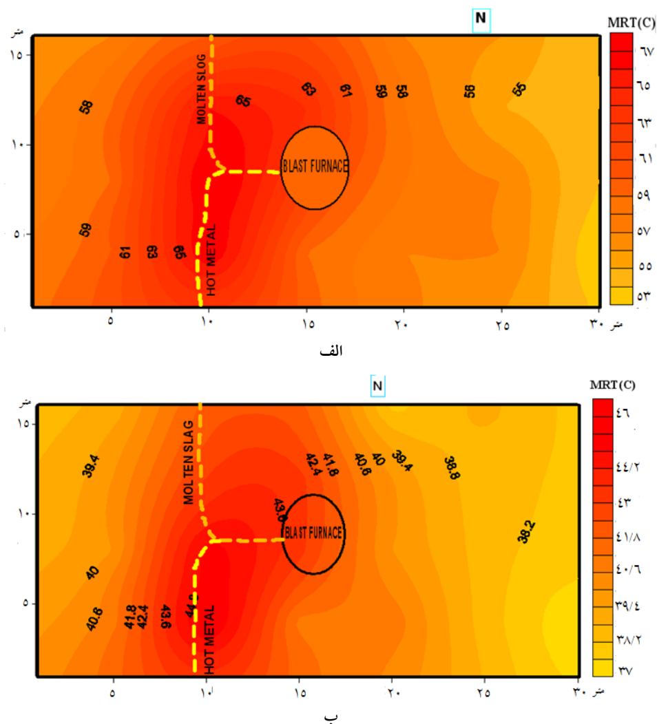
شکل ۳- توزیع حرارتی محوطه کوره بر مبنای دمای تابشی قبل (الف) و بعد (ب) از اجرای مداخلات
