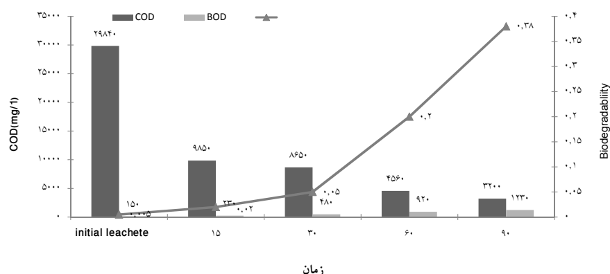
شکل ۶: تغییرات نسبت BOD_5/COD (قابلیت تجزیه پذیری بیولوژیکی) و افزایش راندمان تصفیه شیرابه طی زمان های مختلف pH=3 و نسبت [Fe^{2+}]=1.14 \text{ mmol/l} : [H_2O_2] را نشان می دهد.
