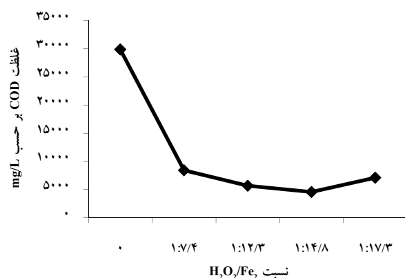
شکل ۲: میزان کاهش COD در نسبت‌های مختلف Time=۶۰ min, PH=۳, H 2 O 2 /Fe ۲+
