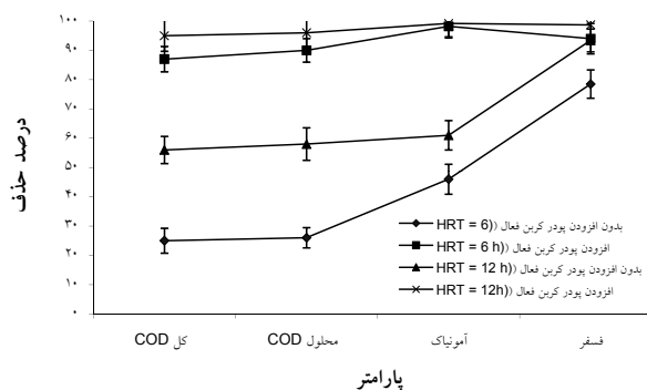
شکل ۳: مقایسه بازده حذف پارامترهای مورد بررسی در شرایط راهبری مختلف
