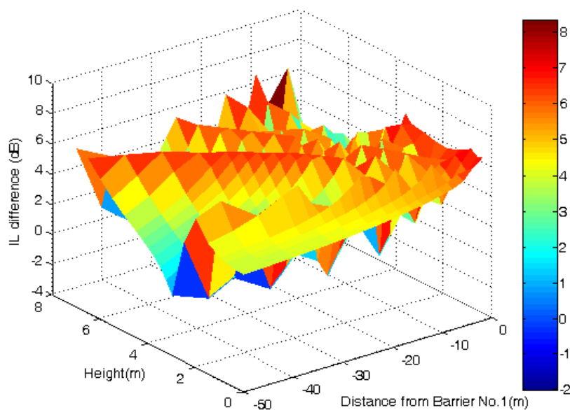
شکل ۹- میزان تغییر در افت صدا در فرکانس ۵۰۰ هرتز در مانع مدل PG نسبت به مانع مدل PAAT در میدان وسیعی
