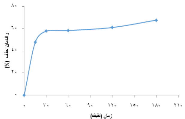
نمودار ۲- اثر زمان تماس بر ظرفیت جذب کروم شش ظرفیتی توسط جاذب خاکستر ساقه زرشک (غلظت اولیه کروم = ۲ میلی گرم بر لیتر)
