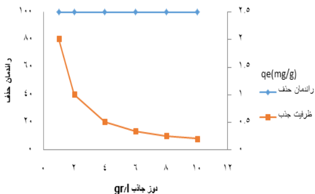
نمودار ۲- اثر دوز جاذب بر راندمان جذب کروم شش ظرفیتی توسط جاذب خاکستر ساقه زرشک (غلظت اولیه کروم = ۲ میلی گرم بر لیتر)
