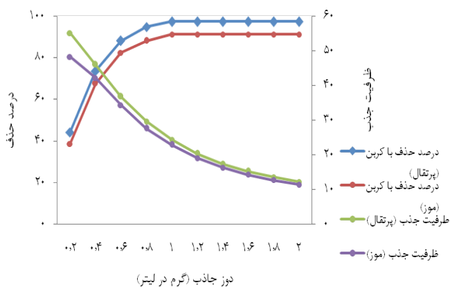
نمودار ۵. تأثیر دوز جاذب بر روی کارایی حذف (غلظت ۲-کلروفنل ۲۵ میلی‌گرم در لیتر، زمان تماس ۶۰ دقیقه، PH=5 )
