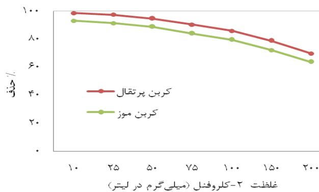
نمودار ۲. تأثیر دوز جاذب بر روی کارایی حذف ۲-کلروفنل بر روی کارایی حذف (دوز جاذب ۱ گرم در لیتر، زمان تماس ۶۰ دقیقه، PH=5 )
