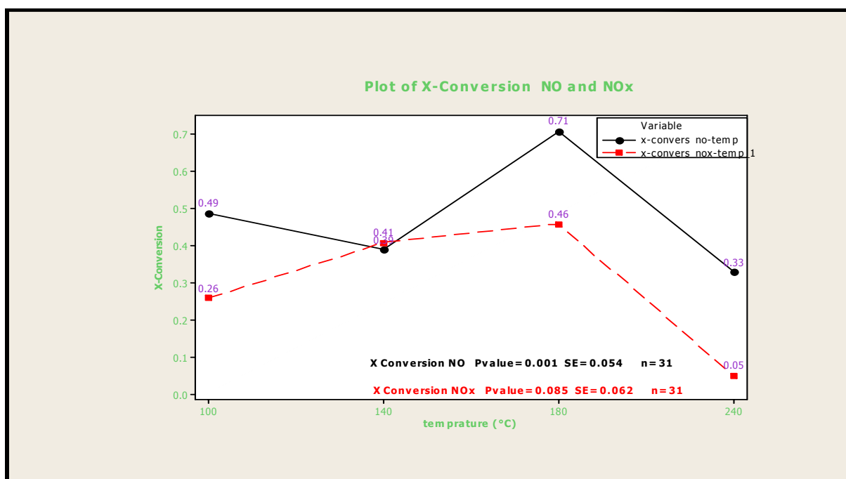
نمودار ۴- پیش بینی روند تاثیر درجه حرارت دردمای بالاتر از ۱۸۰ °C بر ضریب تبدیل NO و NOx در راکتور پلاسما
