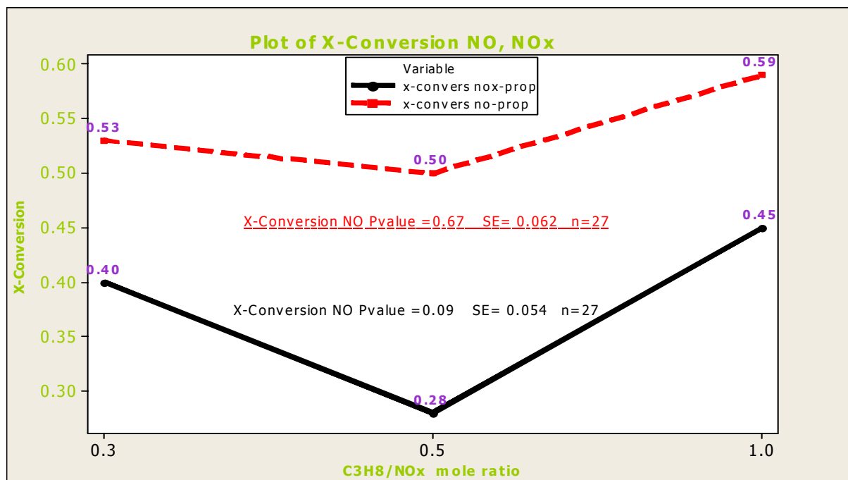
نمودار ۳- روند تاثیر نسبت مولی پروپان بر ضریب تبدیل NO و NOx در راکتور پلاسما
