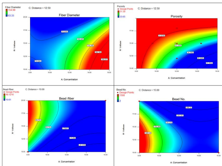
شکل ۱- پلات کنوری از تاثیر همزمان غلظت و ولتاژ در فاصله الکتروریسی معین بر متغیرهای پاسخ
