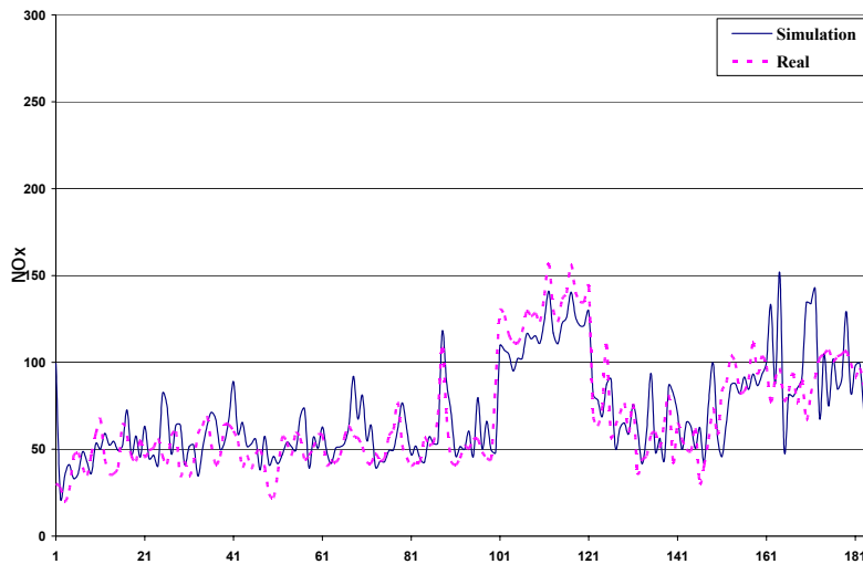
نمودار ۶- مقایسه غلظت NO_x مشاهده شده با مقادیر شبیه سازی شده با استفاده از داده های کالیبراسیون
