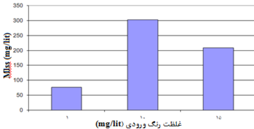
نمودار ۸- مقایسه تغییرات MLSS در راکتور MBBR در غلظت های رنگ ورودی ۱، ۱۰ و ۱۵ میلی گرم در لیتر و COD = 1000\text{mg/l}
