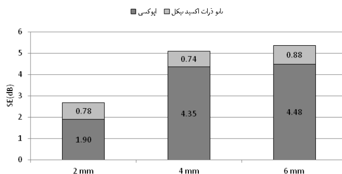
نمودار ۳- سهم فیلر و ماتریس در بر اثربخشی حفاظتی سپرهای نانوکامپوزیتی (بر حسب دسی بل)
