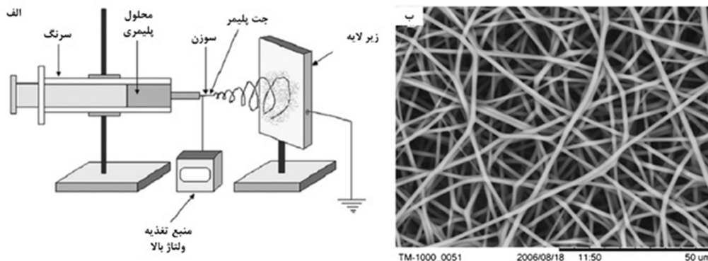
شکل ۱- الف) دستگاه استاندارد الکتروروسی و ب) تصویر میکروسکوپ الکترونی روبشی از نانوالیاف پلی اورتان الکتروروسی شده (۶)
