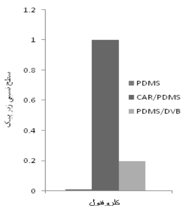
شکل ۱- میزان نسبی بازیافت ۲-کلروفنول از روی فیبرهای PDMS 100µm، CAR/PDMS 75µm و PDMS/DVB µm 65 در حالت تماس یافته خارج از غلاف
