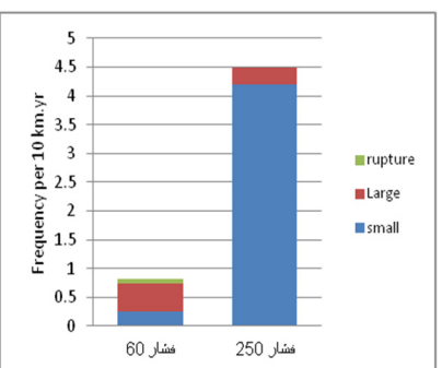
شکل ۶- ارتباط بین سائز نشت و فشار شبکه توزیع شکل ۷- نحوه کشف و گزارش نشت
