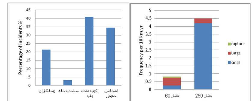
شکل ۶- ارتباط بین سائز نشت و فشار شبکه توزیع شکل ۷- نحوه کشف و گزارش نشت
