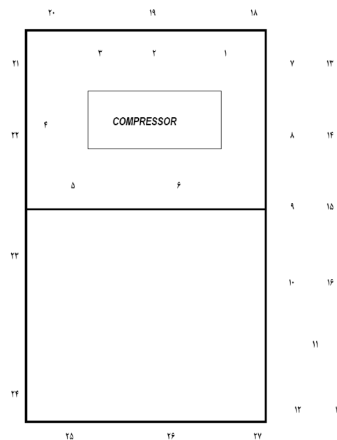
شکل ۱- موقعیت نقاط اندازه‌گیری پیرامون کمپرسور (در حالت خاموش)
