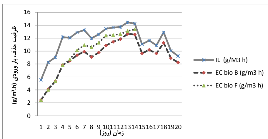
شکل (۳)- تغییرات ظرفیت حذف (EC) بیوفیلتر باکتریایی و قارچی نسبت به میزان ورودی آلاینده تولوئن (LR) به ترتیب طی ۲۰ و ۱۴ روز عملیات. IL: میزان بار ورودی، EC bio B: ظرفیت حذف بیوفیلتر باکتریایی، EC bio F: ظرفیت حذف بیوفیلتر قارچی
