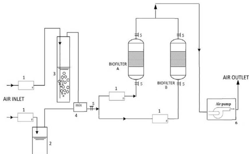
شکل (۱) - شماتیکی از ستاپ آزمایش (بیوفیلتر باکتریایی و بیوفیلتر قارچی)، ۱. روتامتر، ۲. ایمپینجر حاوی تولوئن خالص، ۳. ستون پیش مرطوب ساز، ۴. اتاقک اختلاط، ۵. پورت های نمونه برداری از جریان هوا، ۶. هواکش دور متغیر
