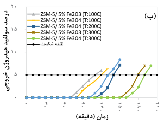
شکل ۵: (الف) منحنی شکست بسترهای کاتالیستی با درصدهای بارگذاری مختلف نانو ذرات آهن (دما: 200^{\circ}C - دبی (lit/min) - غلظت: 60\text{ ppm} ). (ب) منحنی شکست بسترهای کاتالیستی در دماهای مختلف راکتور (دما: 200, 300, 100^{\circ}C - دبی (lit/min) - غلظت: 60\text{ ppm} ). (ج) ظرفیت جذب بسترهای کاتالیستی با درصد بهینه بارگذاری نانو ذرات آهن و دمای بهینه (دما: 300^{\circ}C - دبی (lit/min) - غلظت: 30-60-90-120\text{ ppm} ).
