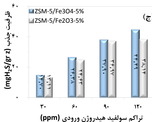
شکل ۵: (الف) منحنی شکست بسترهای کاتالیستی با درصدهای بارگذاری مختلف نانو ذرات آهن (دما: 200^{\circ}C - دبی (lit/min) - غلظت: 60\text{ ppm} ). (ب) منحنی شکست بسترهای کاتالیستی در دماهای مختلف راکتور (دما: 200, 300, 100^{\circ}C - دبی (lit/min) - غلظت: 60\text{ ppm} ). (ج) ظرفیت جذب بسترهای کاتالیستی با درصد بهینه بارگذاری نانو ذرات آهن و دمای بهینه (دما: 300^{\circ}C - دبی (lit/min) - غلظت: 30-60-90-120\text{ ppm} ).
